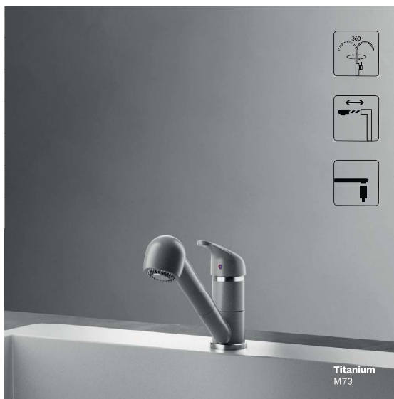
Vienas sviras ūdens maisītājs ar grozāmu snipi un izvelkamu uzgali
