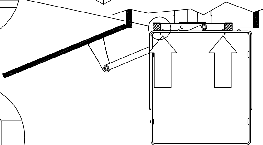
Montaggio Anta Sinistra Left-Hand door mounting
